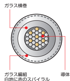
断面図
